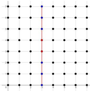
Schéma 14 : droite parallèle à l'axe des ordonnées
