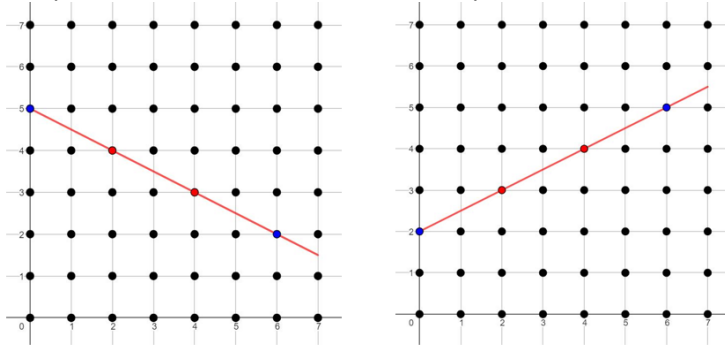
Schéma 15 : passage au symétrique pour a < 0
