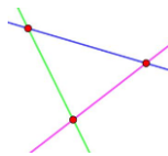
Schéma 6 a : les trois droites formés
