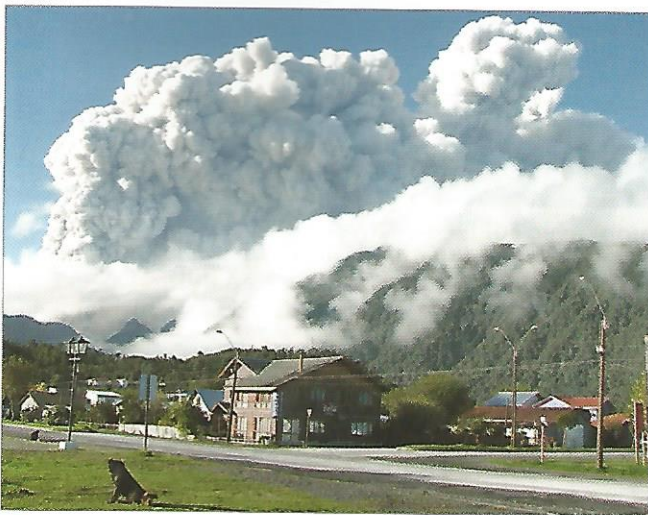
c Nuée ardente au Chili, en juin 2008.
