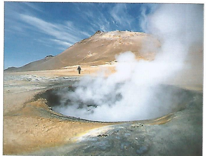
d Fumerolles en Islande.
