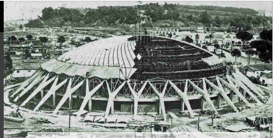
P. Luigi Nervi et A. Vitellozzi, Petit Palais des sports, 1958-1959, Rome
