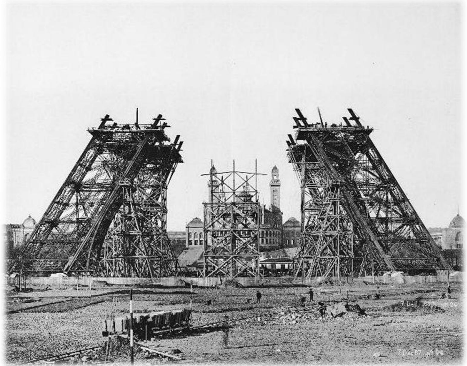
Montage de la partie inférieure sur les pylônes en charpente
